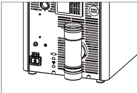
Raccordement conduit de fumée - version standard
