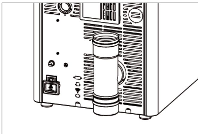
Uitlaataansluiting - standaarduitvoering
