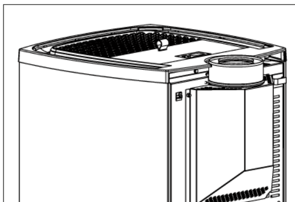
Raccordement conduit de fumée - version coaxiale
