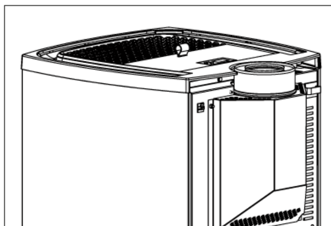
Uitlaataansluiting – coaxiale uitvoering
